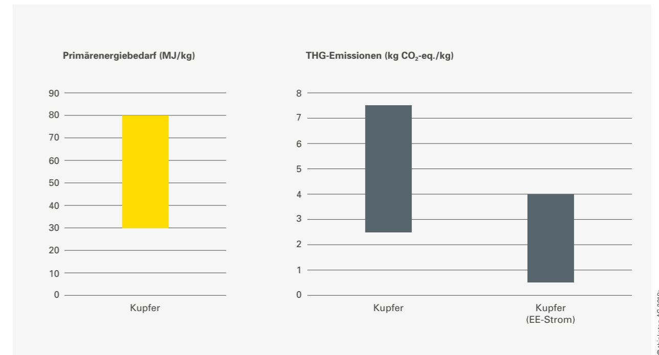
Abbildung 7-6: Primärenergiebedarf und THG-Emissionen infolge der Bereitstellung von 1 kg Kupfer
