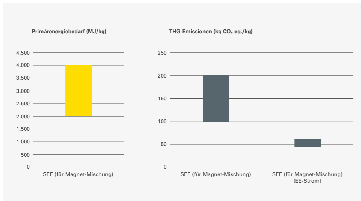
Abbildung 7-5: Primärenergiebedarf und THG-Emissionen infolge der Bereitstellung von 1 kg SEE (für Magnet-Mischung)
