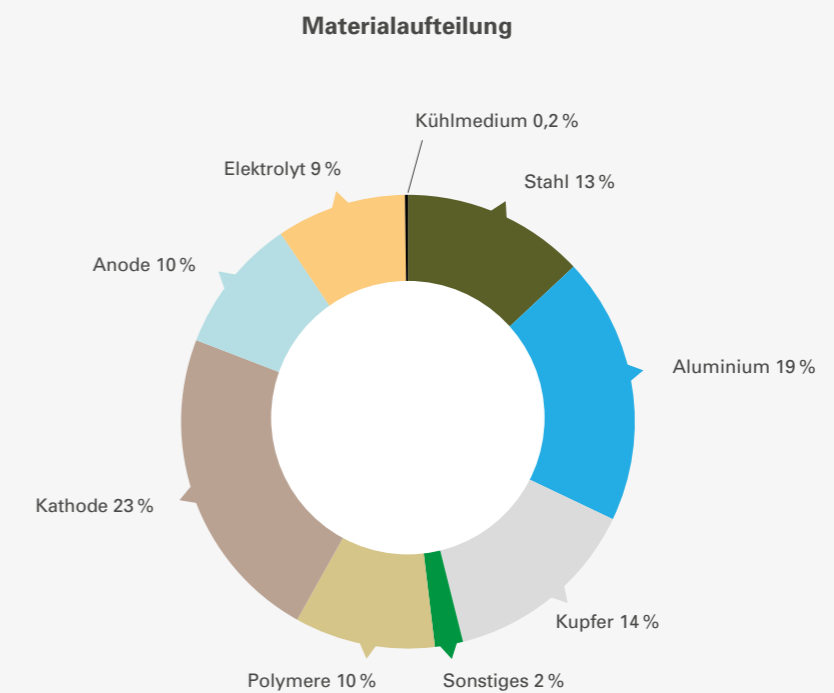
Abbildung 10-1: Typische Anteile von Komponenten (oben) und Materialien (unten) in der Batterie eines BEV
